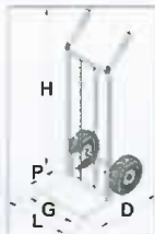
MOD. 131M195 PORTATA Kg 100 PESO Kg 9,8 RUOTE PIENE Ø 175 L= 540 D=360 H=930 G=380 P=190
